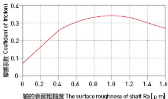
图表 HPP13-6: 摩擦系数与轴表面粗糙度关系图表
