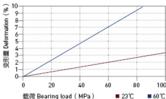
图表 HPP13-3: 载荷 - 温度图表
