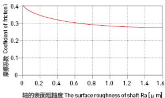
图表 HPP21-6: 摩擦系数与轴表面粗糙度关系图表
