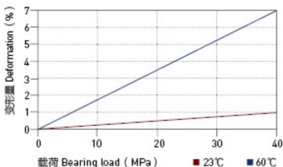
图表 HPP21-3: 载荷 - 温度图表
