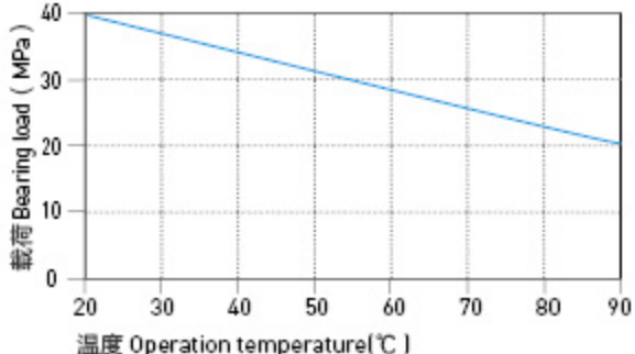
图表 HPP21-3: 载荷 - 温度图表
