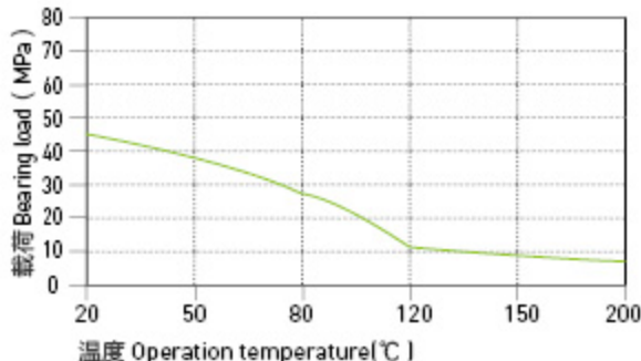
图表 HPP24-3: 载荷 - 温度图表
