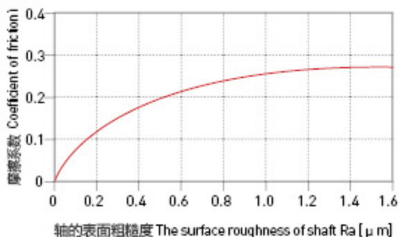
图表 HPP24-6: 摩擦系数与轴的表面粗糙度关系图表
