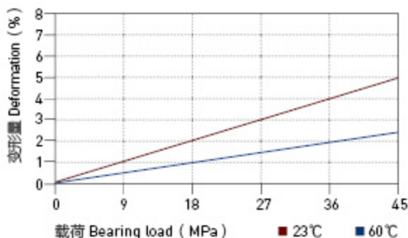
图表 HPP24-3: 载荷 - 温度图表
