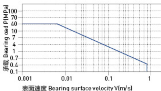
图表 HPP24-1: PV 图表
